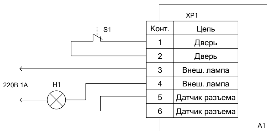
Рис. 3. Схема подключения цепей блокировки и внешней сигнализации.
